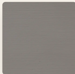
Doleriet
